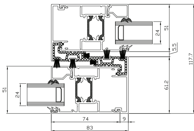
Snitt skjøt dører
